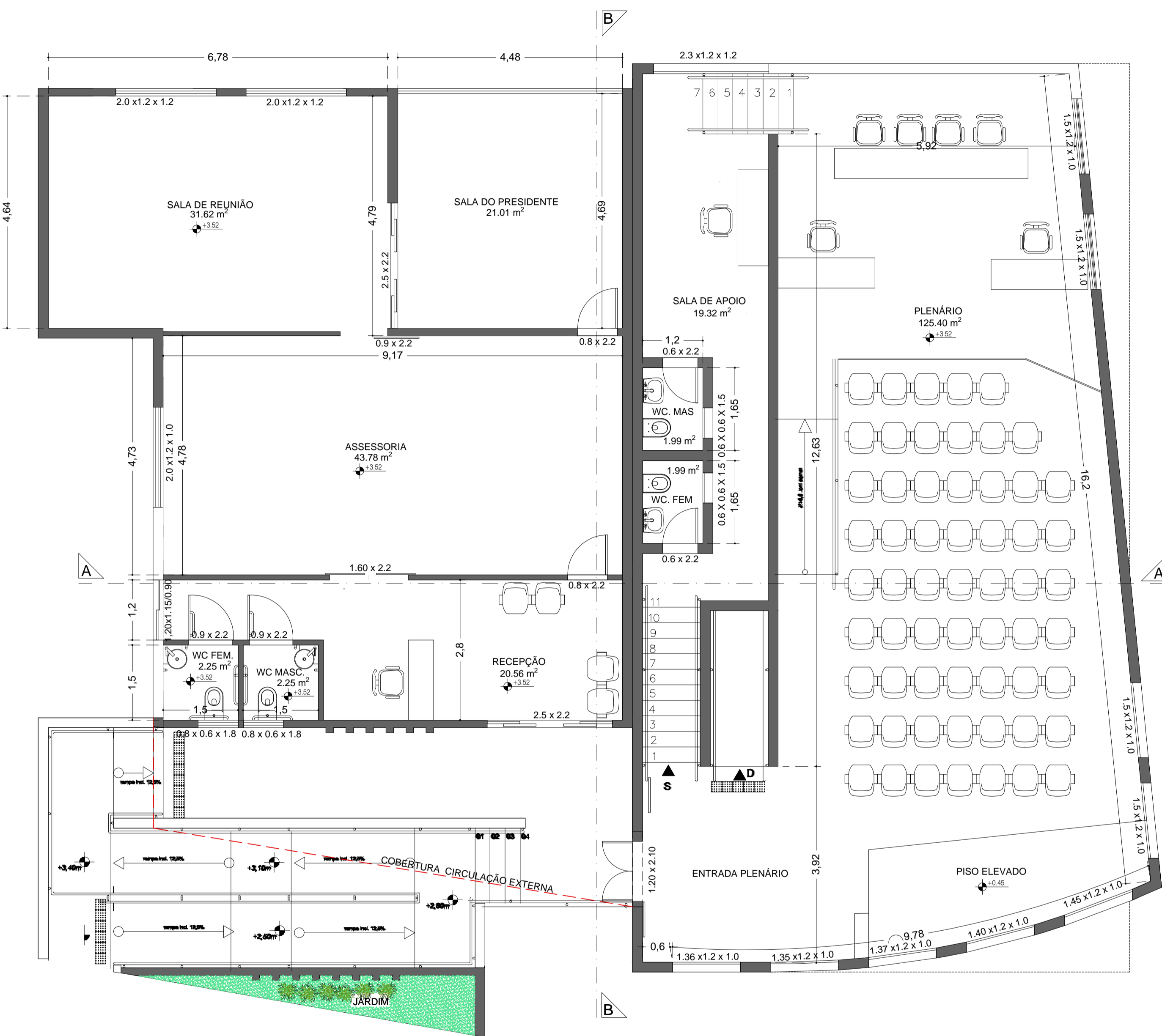
PLANTA PAVIMENTO SUPERIOR - ESC. 1/100
