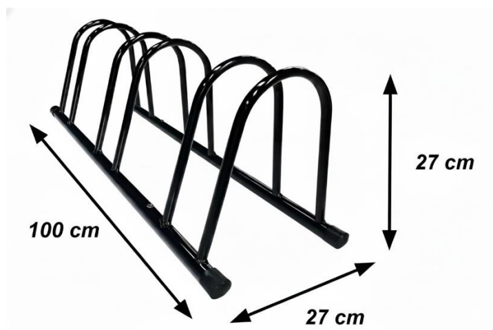
Figura 03 – Modelo do bicicletário.
