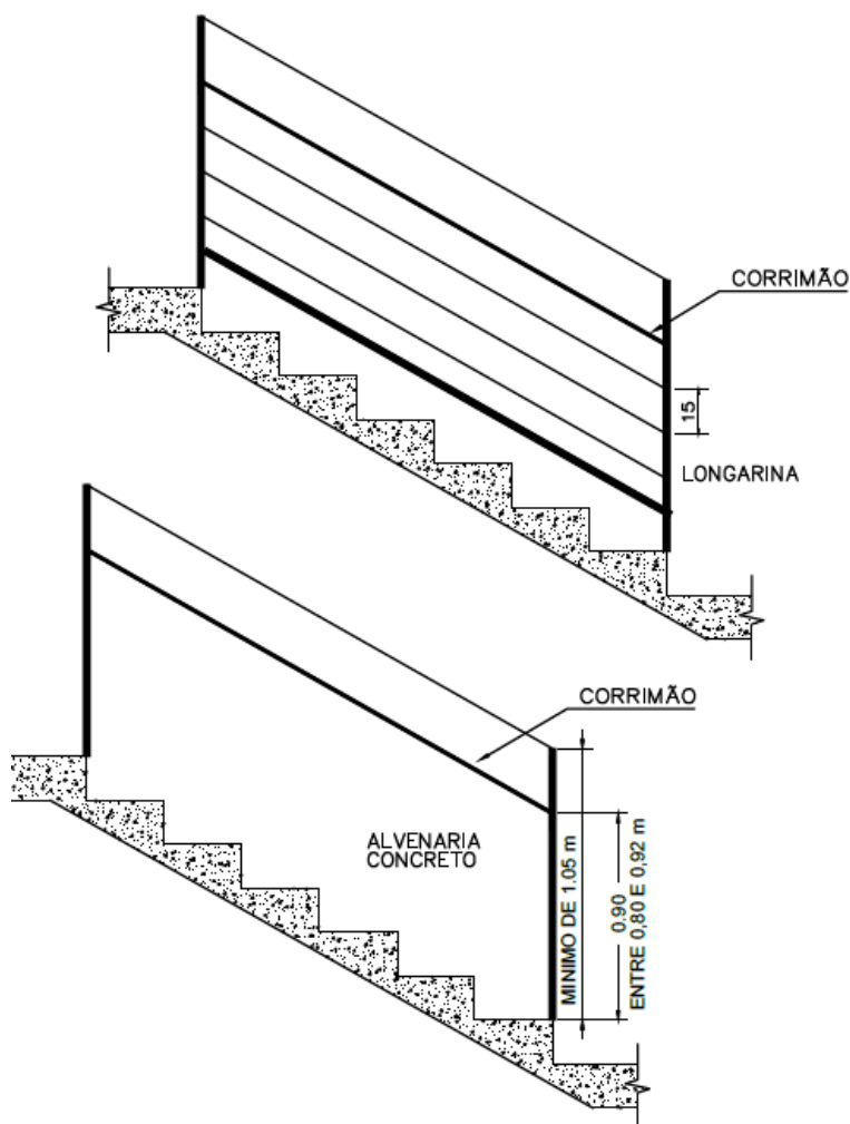
Figura 01 – Detalhes do corrimão e guarda-corpo.
