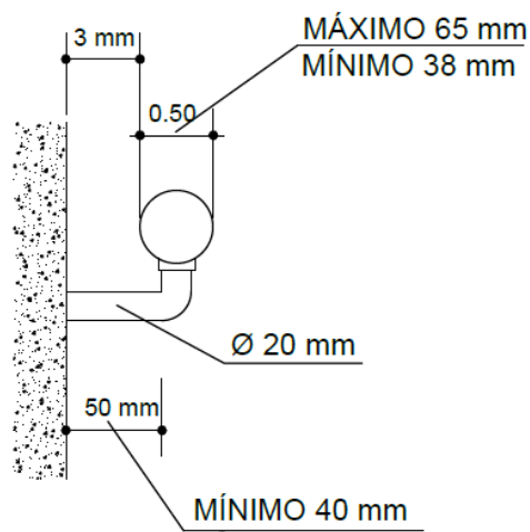
Figura 02 – Detalhes do corrimão.
